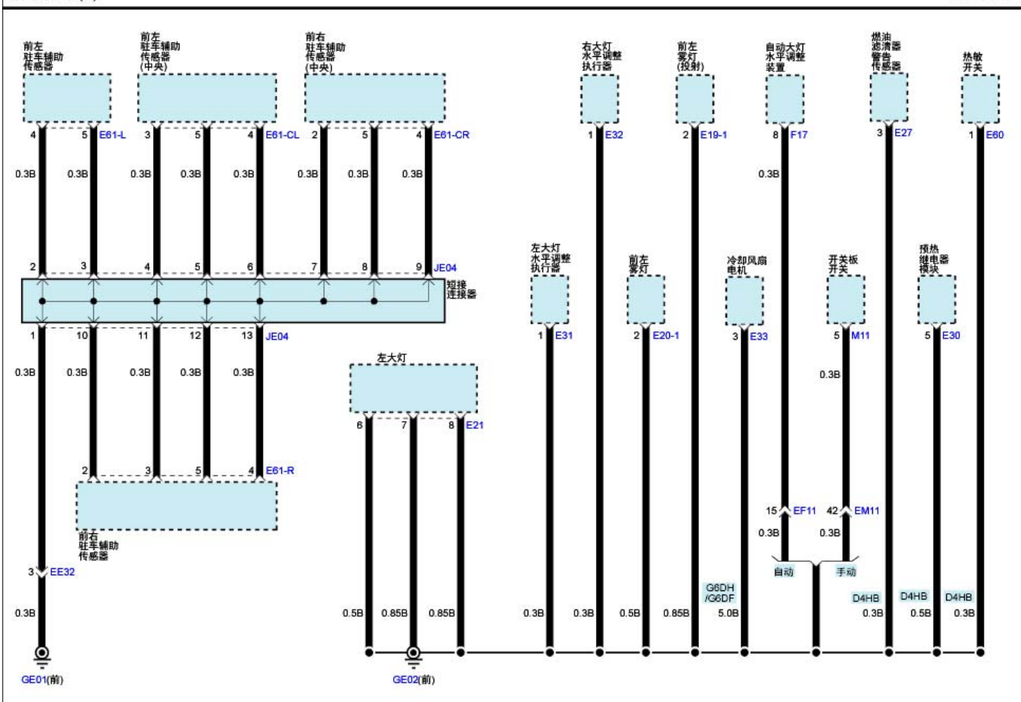
搭铁分布(5)
